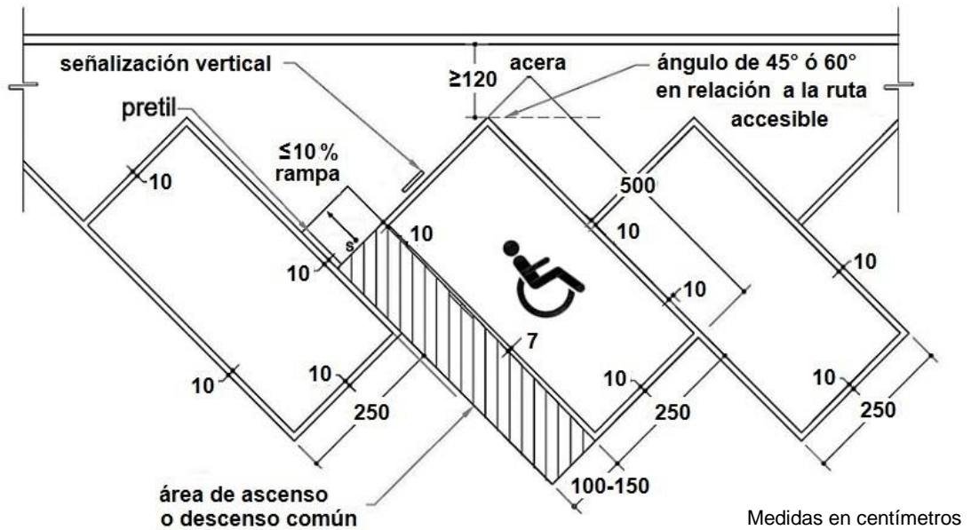
Figura 36 - Planta de un Estacionamiento: Rectángulo oblicuo (a 45^\circ ó 60^\circ en relación a la ruta accesible) delimitado por una franja con espesor de 10 cm conteniendo el símbolo de accesibilidad y la indicación de una rampa próxima a uno de los laterales
